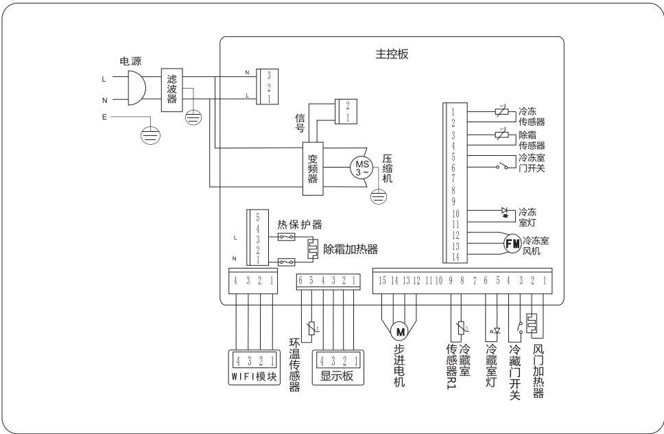
电路图（BCD-516WDBIZW）
